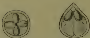
Fig. 25. Zwei Sporen v. Chl. mucronatum , links von oben, rechts von der Seite gesehen.
